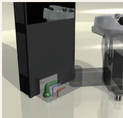
配管カバー内で立ち上げた場合 ※配管カバー床下 (EA-YMS2PY) をお選びください。
